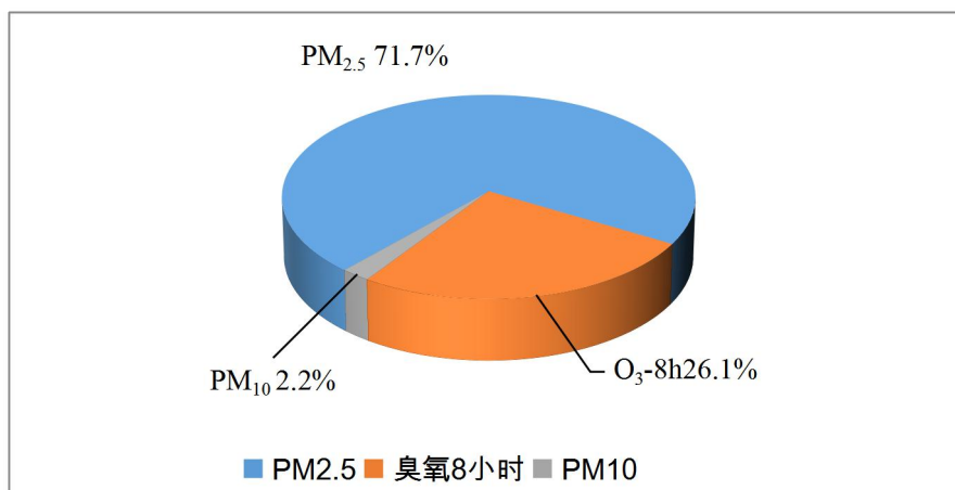
图 4-2 2020 年 46 个污染日中首要污染物占比图
