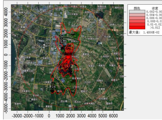
NOx 日平均浓度贡献值
