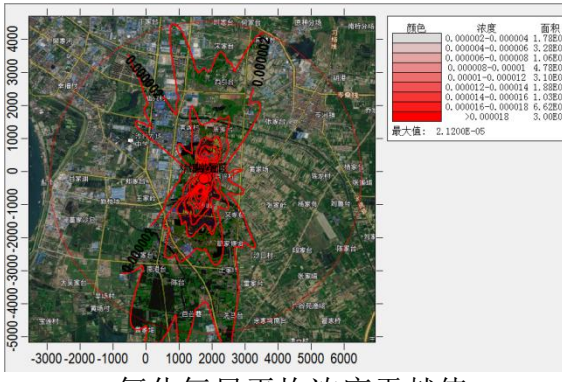
氯化氢日平均浓度贡献值
