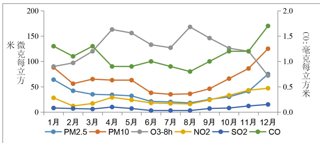
图 4-4 2020 年荆州中心城区 6 项污染物月均浓度变化图
