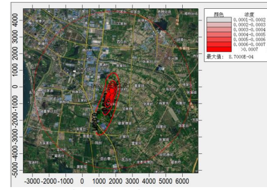
CO 年平均浓度贡献值
