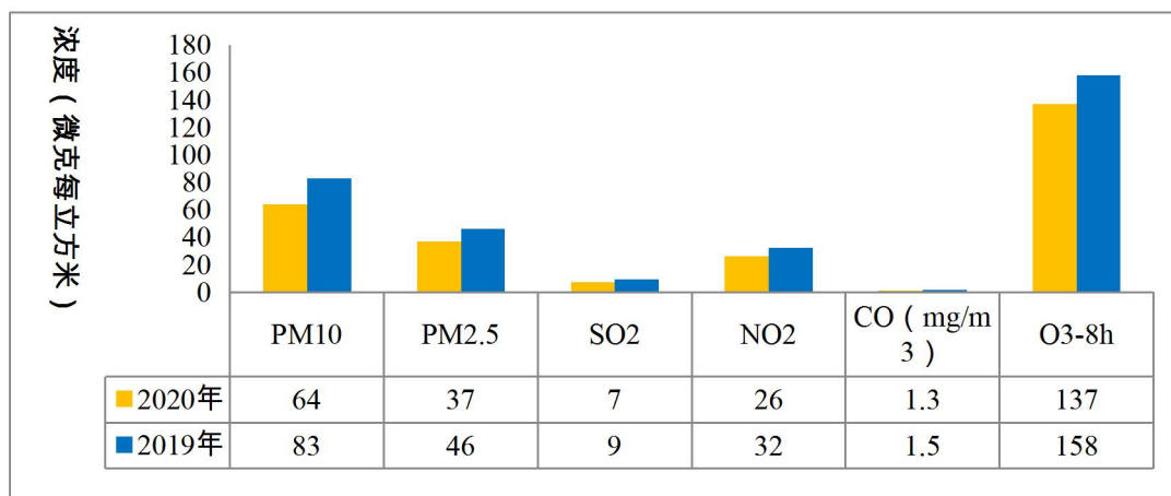
图 4-3 2020 年荆州中心城区 6 项污染物与 2019 年对比图
