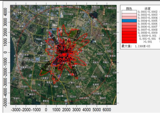
SO 2 1 小时浓度贡献值
