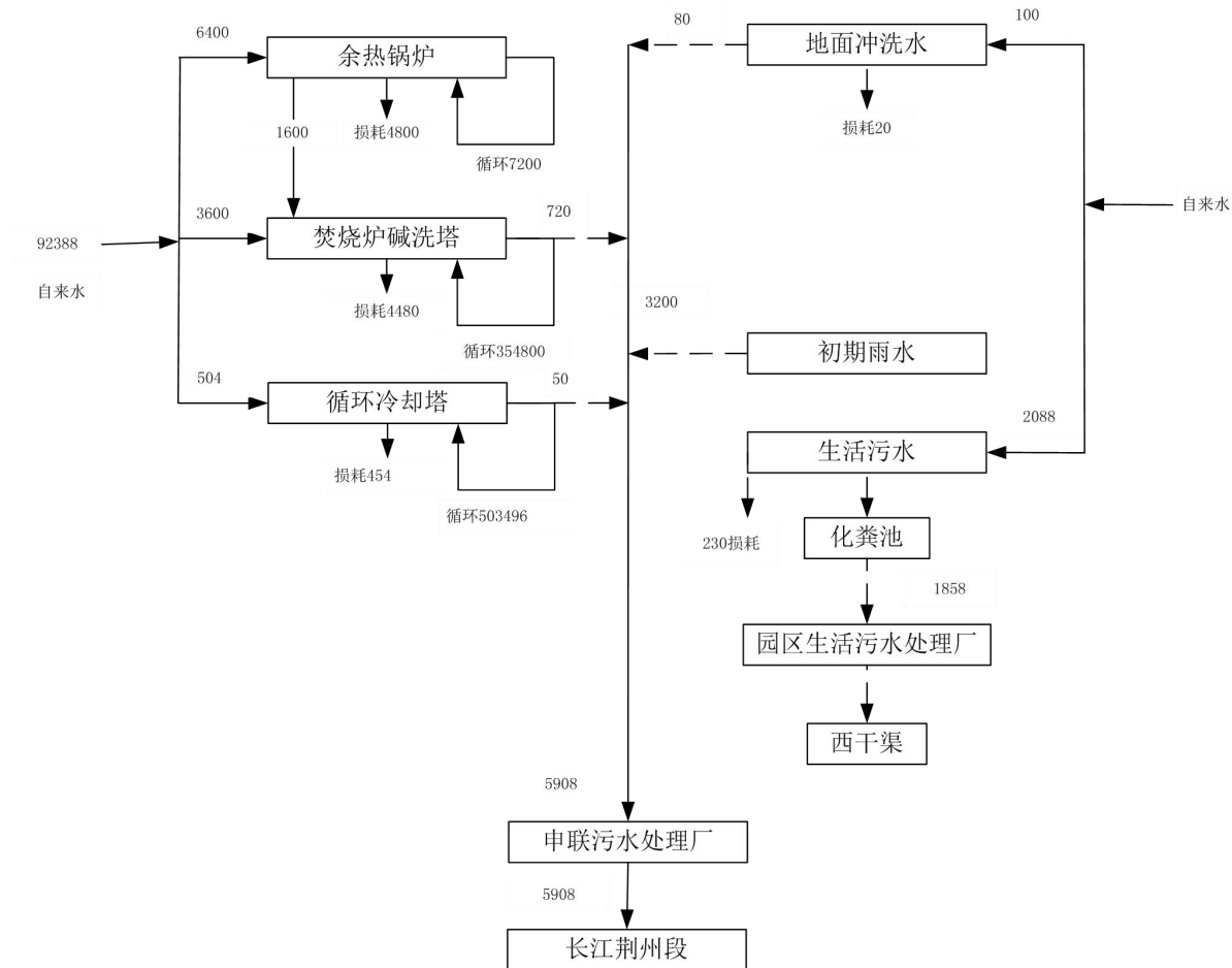
图 3-1 水平衡示意图 (单位: m³/a)
