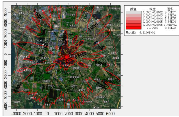
二噁英非正常工况 1 小时浓度贡献值
