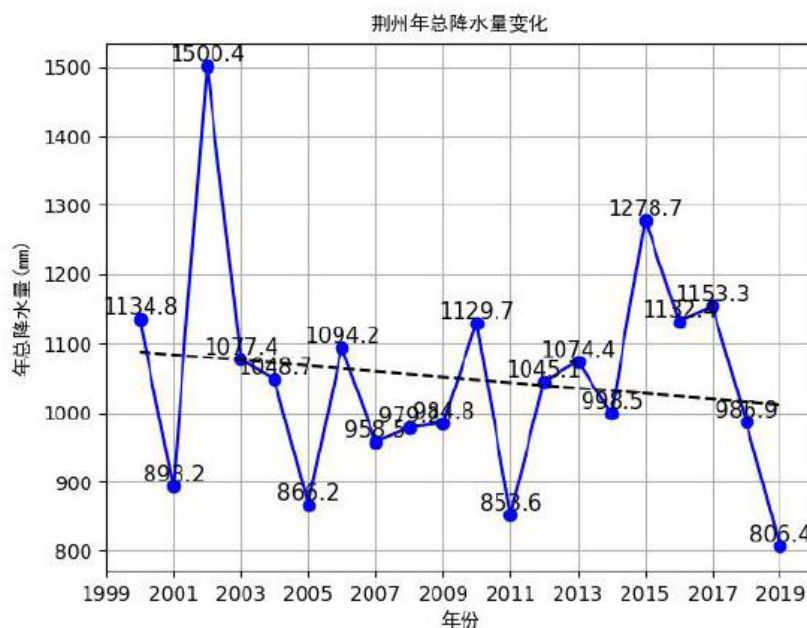
图 5-6 荆州（2000-2019）年总降水量（单位：毫米，虚线为趋势线）
