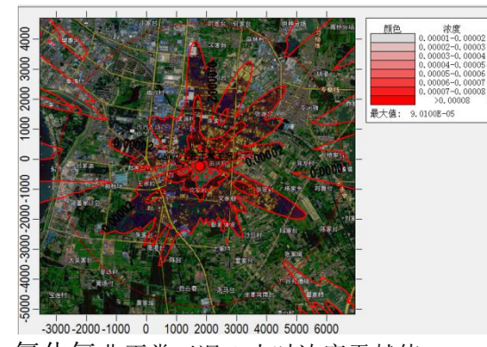
氯化氢非正常工况 1 小时浓度贡献值
