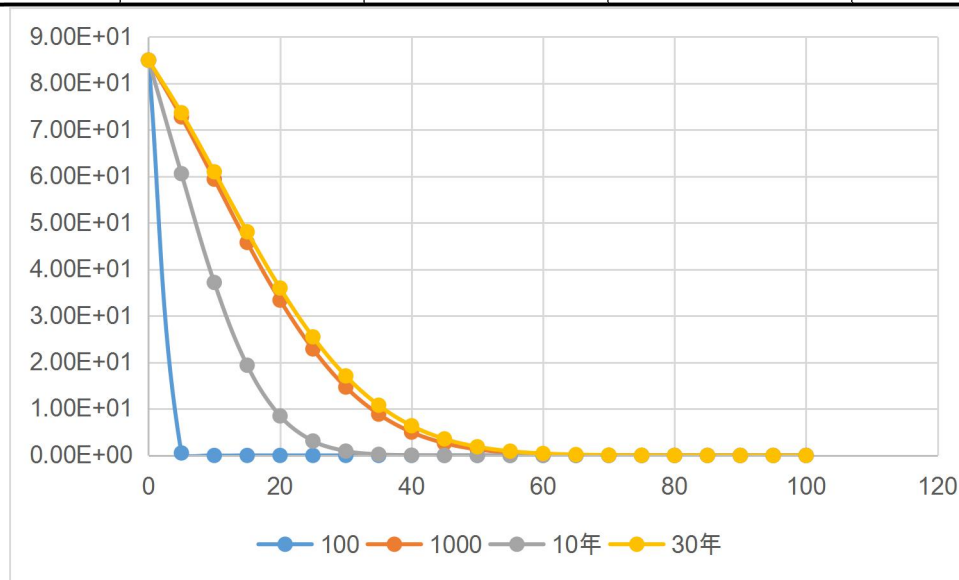
图 6-3 连续泄露耗氧量污染扩散距离图
