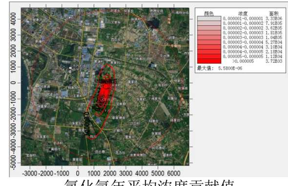
氯化氢年平均浓度贡献值
