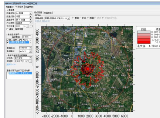
TVOC 非正常工况 1 小时浓度贡献值
