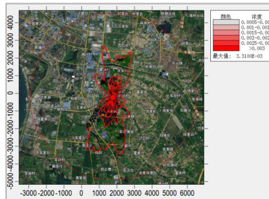
CO 日平均浓度贡献值
