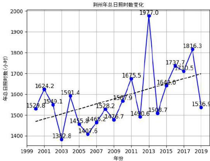
图 5-8 荆州（2000-2019）年日照时长（单位：小时，虚线为趋势线）
