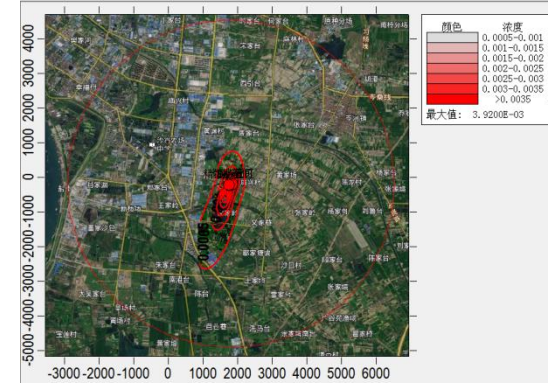
NOx 年平均浓度贡献值
