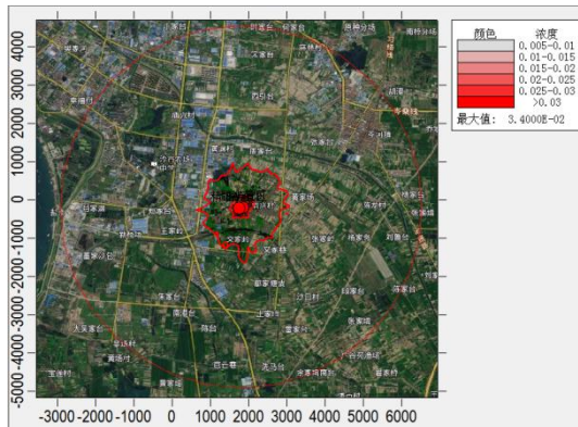
PM 10 1 小时浓度贡献值
