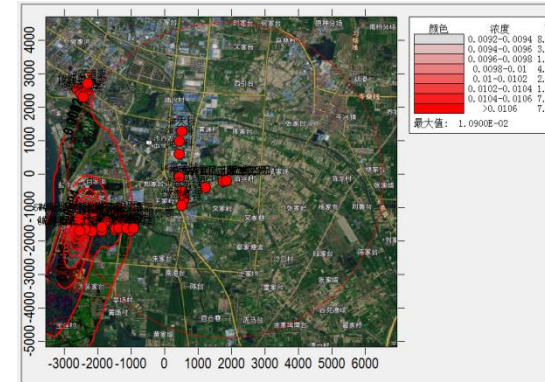
SO 2 年平均浓度叠加预测值
