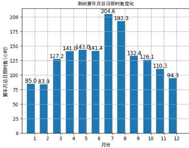
图 5-7 荆州月日照时数（单位：小时）
