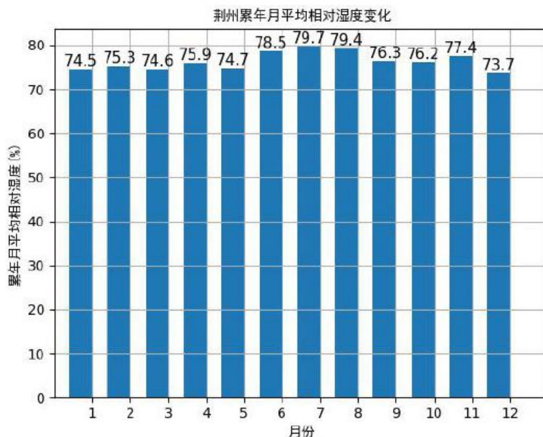
图 5-9 荆州月平均相对湿度（纵轴为百分比）
