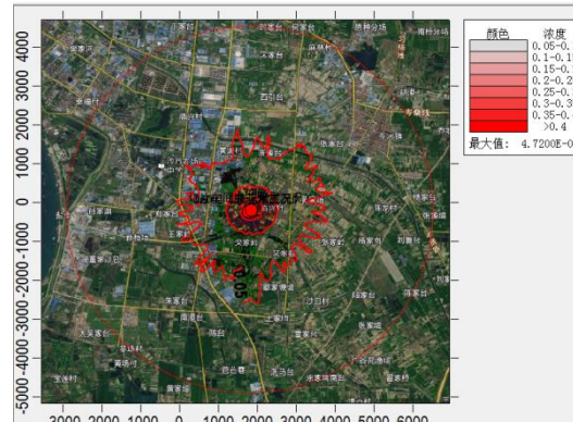
PM 10 非正常工况 1 小时浓度贡献值
