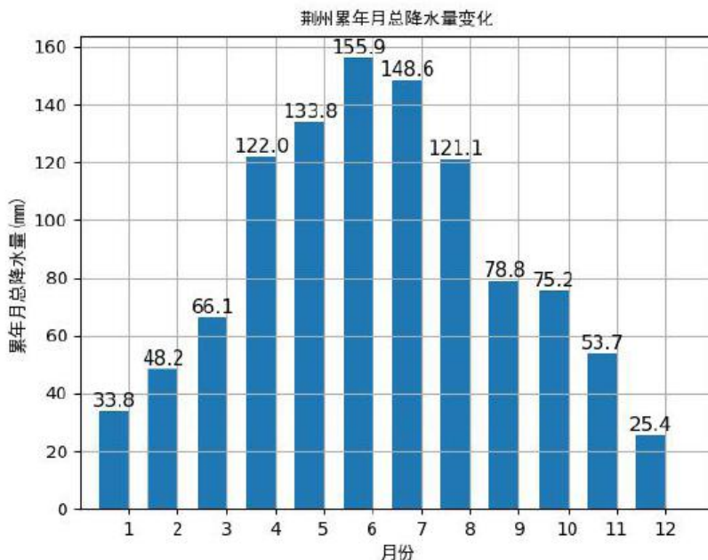
图 6-1 荆州月平均降水量（单位：毫米）
