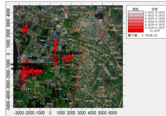
PM 10 年平均浓度叠加预测值
