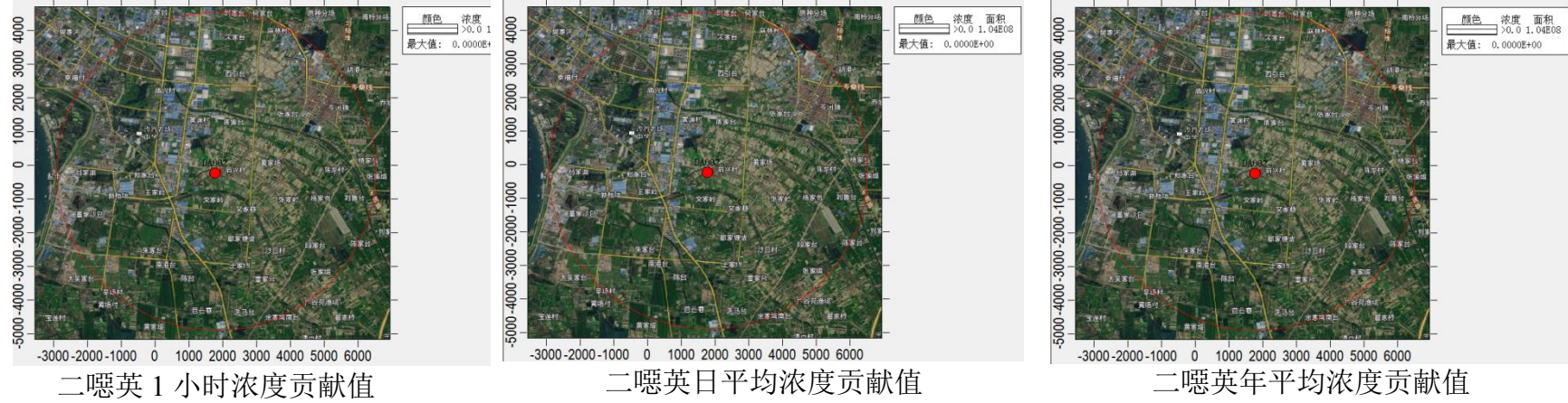
图 5-12 正常工况贡献值预测结果汇总图
